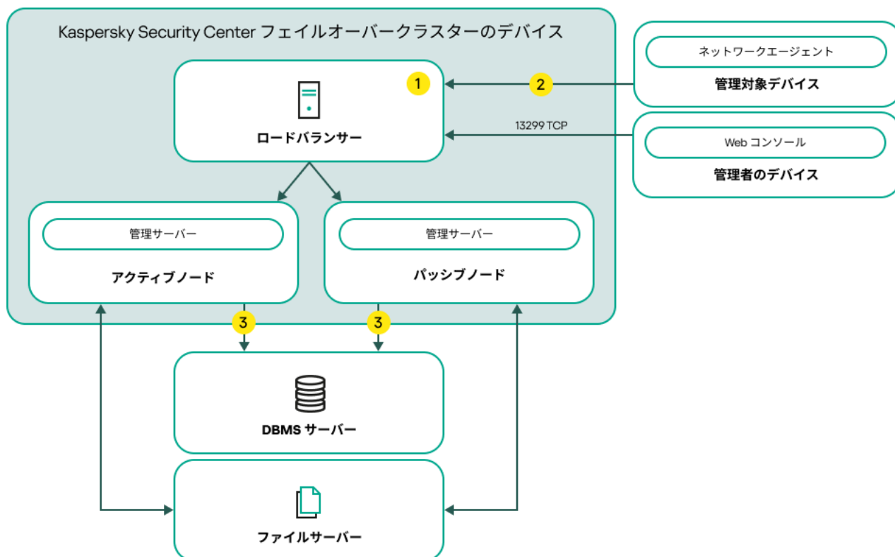
サードパーティのロードバランサーを使用するスキーム
