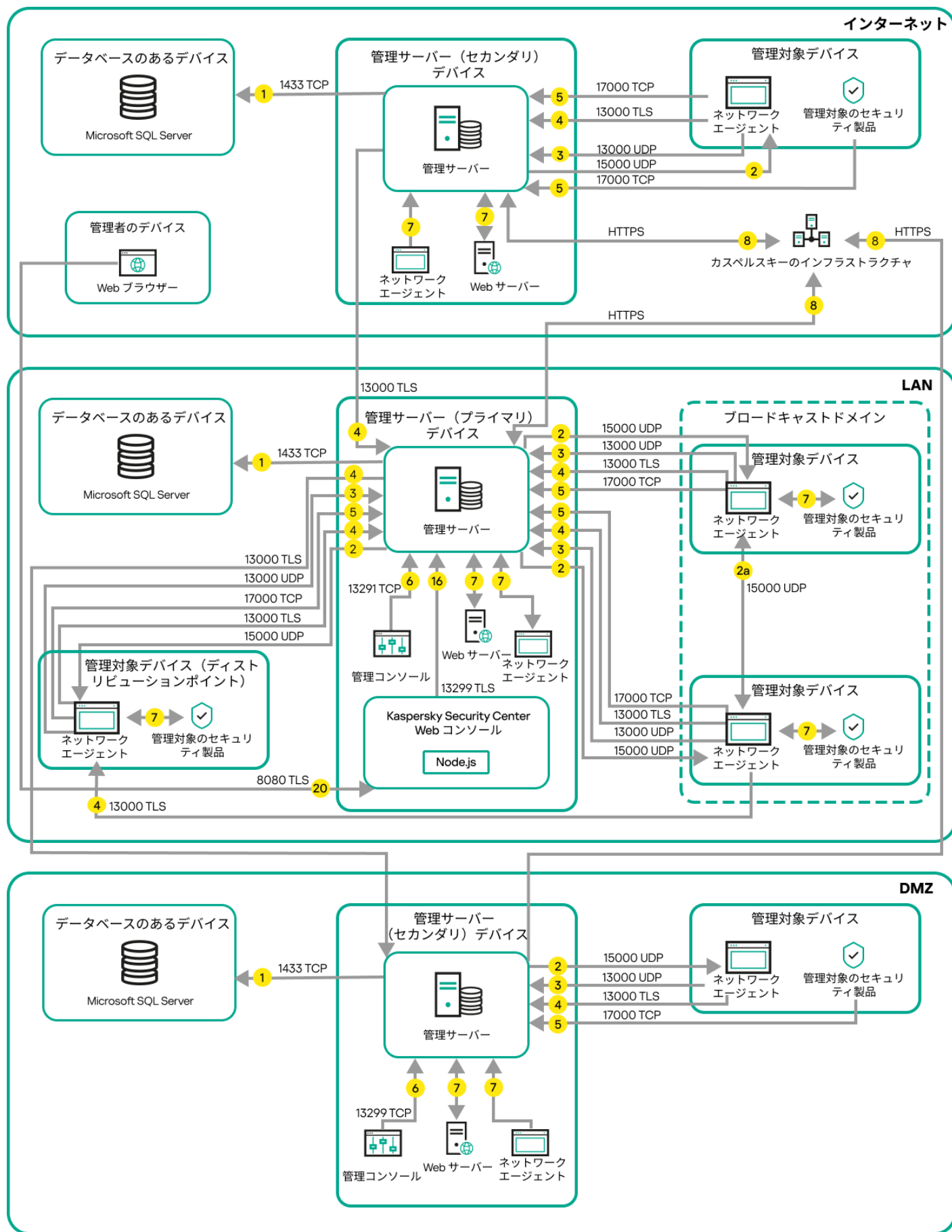
管理サーバの階層構造：プライマリ管理サーバと2台のセカンダリ管理サーバ
