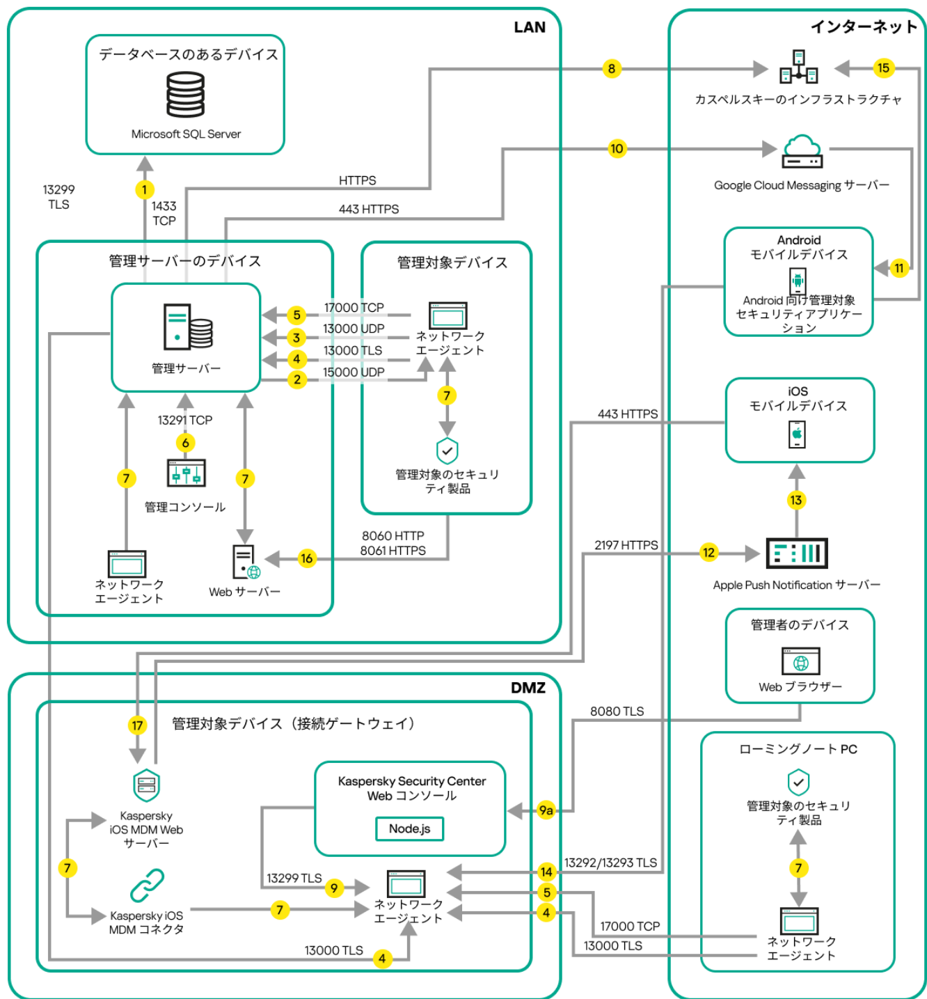
接続ゲートウェイを使用して管理サーバーに接続する管理対象のモバイルデバイス
